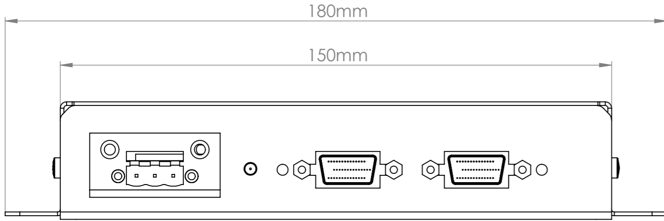
ÖN GÖRÜNÜŞ
